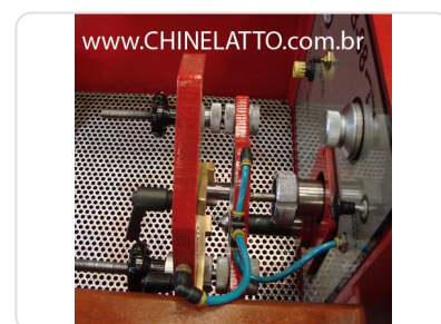
Painel elétrico interno da brunidora de bielas BB-98 com relés e fiação de controle
