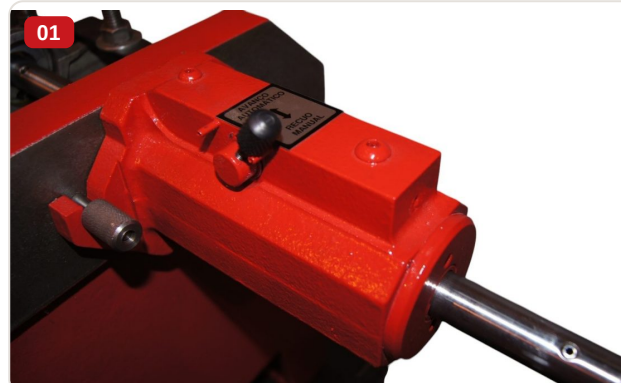
Detalle — Palanca para avance automático o retroceso manual con empuñadura esférica y etiqueta de seguridad
