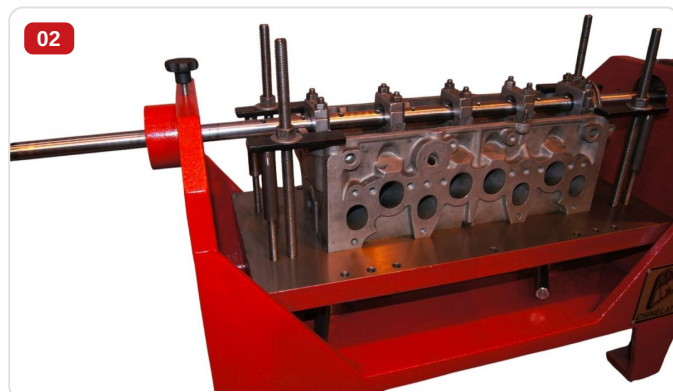
Detalle — Culata automotriz multi-cilindros en aluminio fijada en dispositivo de sujeción para mandrinado de guías de válvulas
