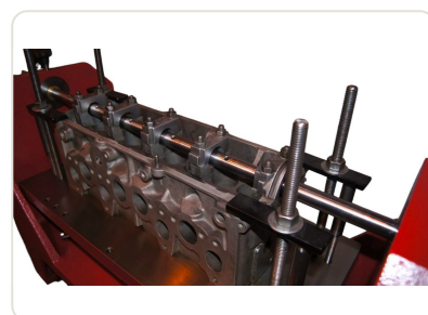
Mandrinadora de Comando de Válvulas EMC-2 Chinelatto — vista en detalle del cabezal con barra portaherramientas
