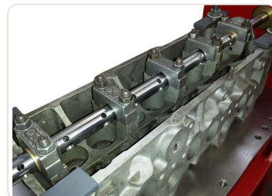
Vista en detalle de la culata automotriz posicionada en la mandrinadora EMC-2 mostrando comando de válvulas y guías de buzos
