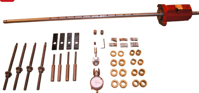
Accesorio normal — Kit completo de la mandrinadora EMC-2 con barra portaherramientas, 40 herramientas de widia, 16 casquillos, reloj comparador, prisioneros y llave Allen
