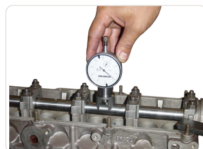
Medición de la altura de la herramienta con reloj comparador DIGIMESS en la mandrinadora EMC-2
