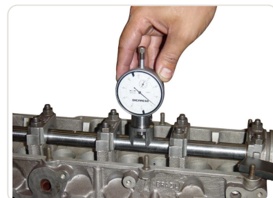
Medição da altura da ferramenta com relógio comparador DIGIMESS na mandrilhadora EMC-2
