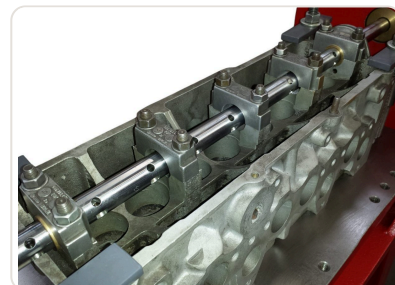
Vista em detalhe do cabeçote automotivo posicionado na mandrilhadora EMC-2 mostrando comando de válvulas e guias dos tuchos
