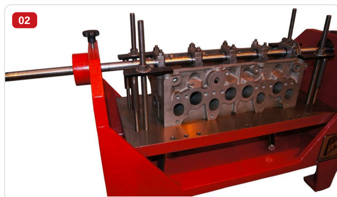
Detalhe — Cabeçote automotivo multi-cilindros em alumínio fixado em dispositivo de aperto para mandrilamento de guias de válvulas
