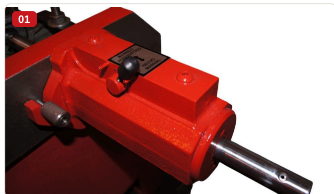
Detalhe — Alavanca para avanço automático ou recuo manual com empunhadura esférica e etiqueta de segurança
