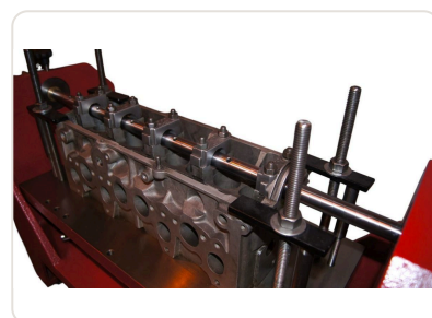
Mandrilhadora de Comando de Válvulas EMC-2 Chinelatto — vista em detalhe do cabeçote com barra porta-ferramenta
