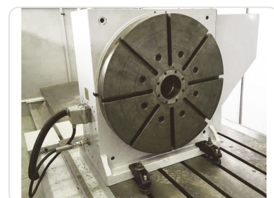
Accesorio opcional — 4º EIXO com servo motor para giros coordenados
