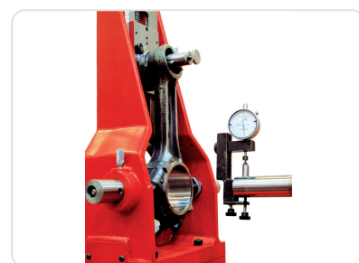
Accesorio normal — Mandrinadora de bielas MB-125 Chinelatto mostrando eje portaherramienta y dispositivo medidor
