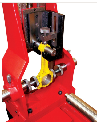
Acessório normal — Dispositivo de fixação amarelo com garras ajustáveis para centragem de bielas na mandrilhadora MB-125
