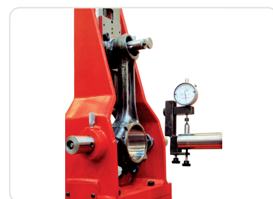
Acessório normal — Mandrilhadora de bielas MB-125 Chinelatto mostrando eixo porta-ferramenta e dispositivo medidor
