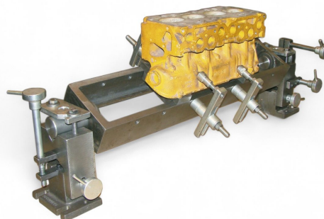
Accesorio opcional — Dispositivo americano para bloques en V y culatas con sistema de fijación ajustable
