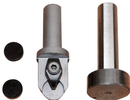
Accesorio opcional — Plaquita CBN (fundición) / PCD (para aluminio) + 1 portaplaquitas + 1 contrapeso para cepillado
