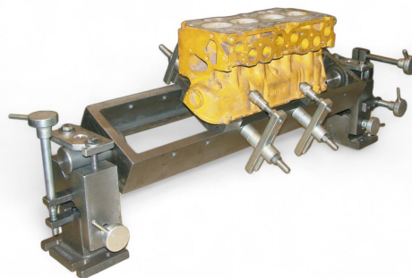
Acessório opcional — Dispositivo Americano para blocos em V e cabeçotes com sistema de fixação ajustável
