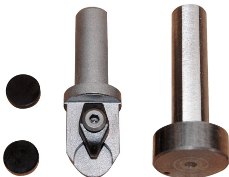
Acessório opcional — Inserto CBN (ferro fundido) / PCD (para alumínio) + 01 porta inserto + 01 contra peso para plainamento
