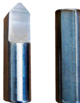
Acessório normal — Ferramenta + contrapeso de aço para plainamento de superfícies planas na plaina PBC-1200X
