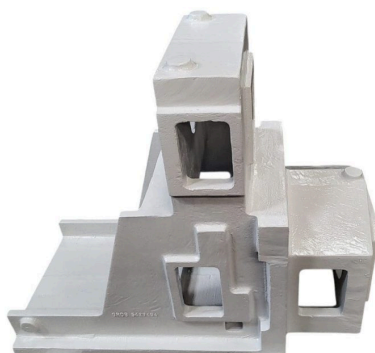
Detalle — 5427493 - 484 kg
