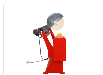
Pulidora de cigüeñal PV-1500 Chinelatto con disco pulidor Ø500mm y motor 3CV para rectificado
