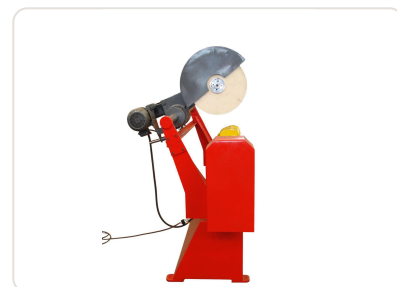
Polidora de virabrequim PV-1500 Chinelatto com disco polidor Ø500mm e motor 3CV para retífica
