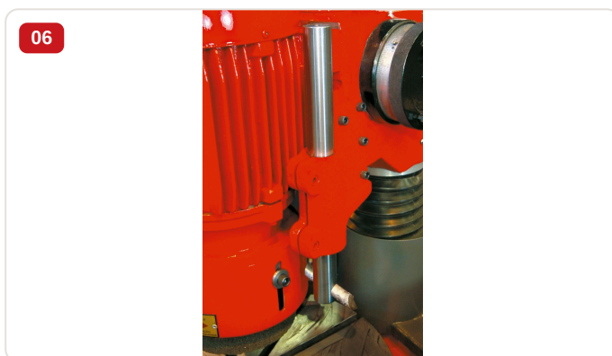
Accesorio normal — Herramienta para romper esquinas en acero en la rectificadora RMG-460X
