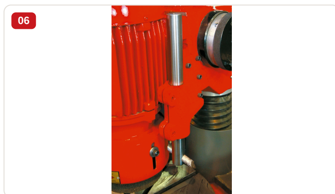
Acessório normal — Ferramenta para quebra de canto em aço na retificadora RMG-460X
