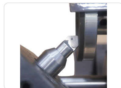
Afilado - Ángulo de salida - Cuchilla Cepilladora
