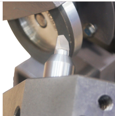
Detalle — Afilado - Herramienta 45 grados - utilización em general
