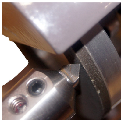
Detalle — Afilado - acabado - Alineadora de bancadas - Rectificadora portatil de cilindros
