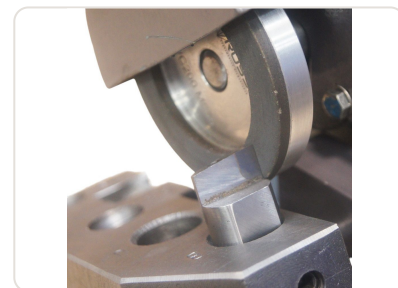
Afilado - Ángulo de ataque - Cuchilla Rectificadora de cilindros de columna
