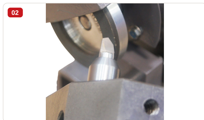
Detalle — Afilado - Herramienta 45 grados - utilización em general
