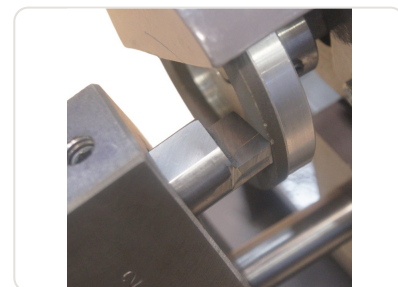
Afilado - Ángulo de lantero - Cuchilla Rectificadora de cilindros de columna
