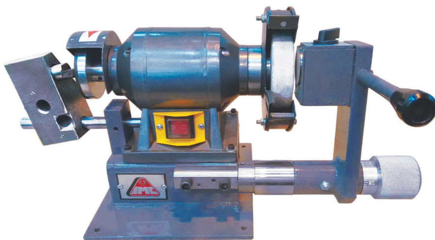
Afiação - Ferramenta Broqueadora de Coluna - Ângulo Ataque
