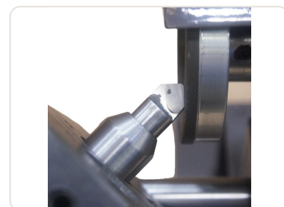
Afiação - Ferramenta Plana - Ângulo Saída
