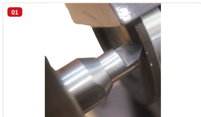
Detalhe — Afição - Ferramenta Plana - Quebra de Canto
