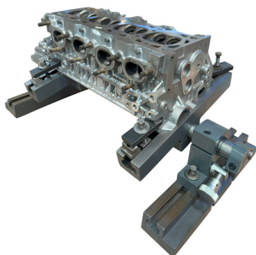
Optional accessory — Image 01 - DI Cradle
