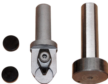
Accesorio opcional — Kit CBN inserto p/ hierro colado
