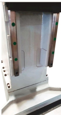
Detalle — Guías lineales en la columna
