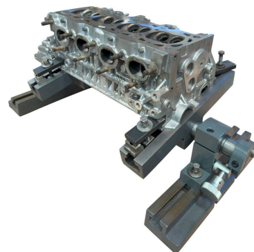
Accesorio opcional — Foto 02 - Dispositivo DI DI p/cabezas con inclinación
