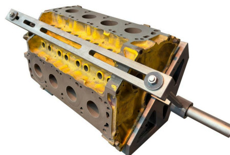
Accesorio opcional — Foto 02 - Dispositivo DB-30°/45° para bloques en "V"
