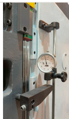
Accesorio normal — 01 Reloj en la columna
