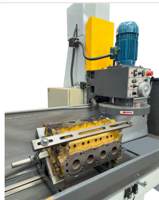
Accesorio opcional — Foto 01 - Dispositivo DB-30°/45° para bloques en "V"
