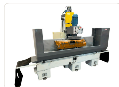
Cepilladora Fresadora de Superficie RSP-1550 Chinelatto para Culatas Automotrices — vista en perspectiva
