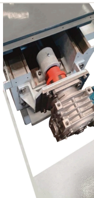
Accesorio normal — Moto-reductor en la mesa
