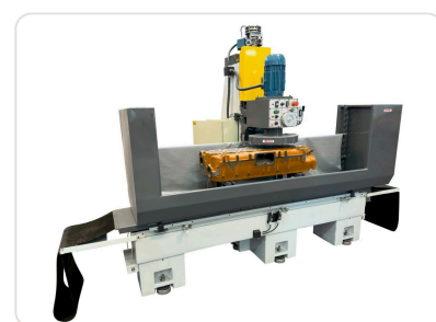
Plaina Fresadora de Superfície RSP-1550 Chinelatto para Cabeçotes Automotivos — vista em perspectiva
