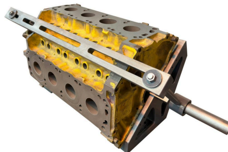
Acessório opcional — Foto 02 - Dispositivo DB-30°/45° para blocos em "V"
