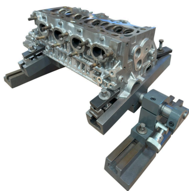
Acessório opcional — Foto 02 - Dispositivo DI para cabeçotes com inclinação
