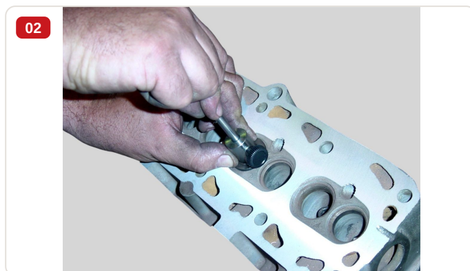
Detalle — Medición con micrómetro de culata de aluminio durante operación de cepillado en rectificadora RV-2
