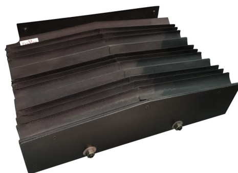
Detalle — Protección acordeón de guías cabezal porta piedra
