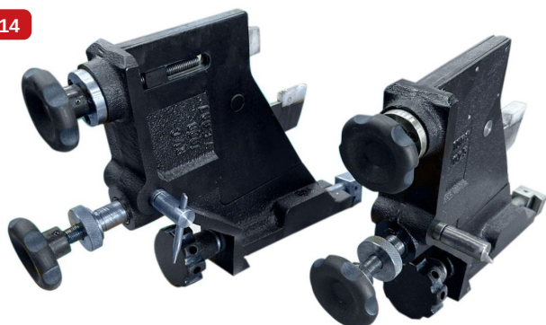
Accesorio normal — 02 Lunetas
