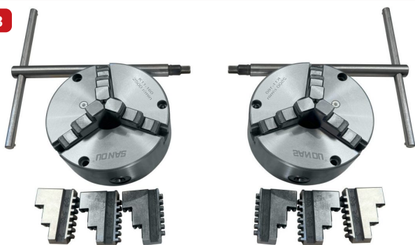
Accesorio normal — 02 chucks Ø8" con mordazas y llaves
