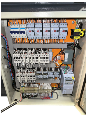
Detalle — Cuadro eléctrico
