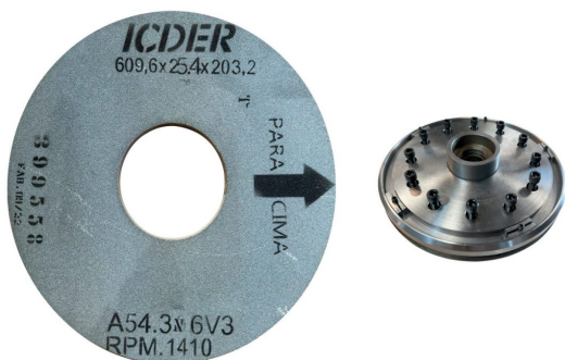
Accesorio normal — Piedra Ø28" x 3/4" con 01 brida
