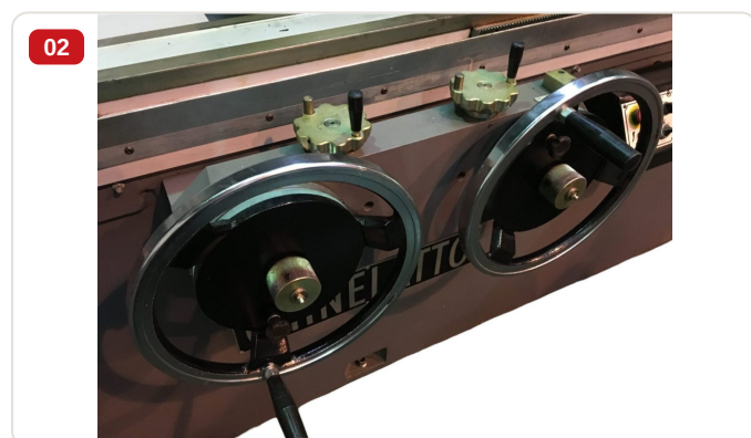
Detalle — Volantes de avance de la mesa y del cabezal del disco en hierro fundido con puños centrales
