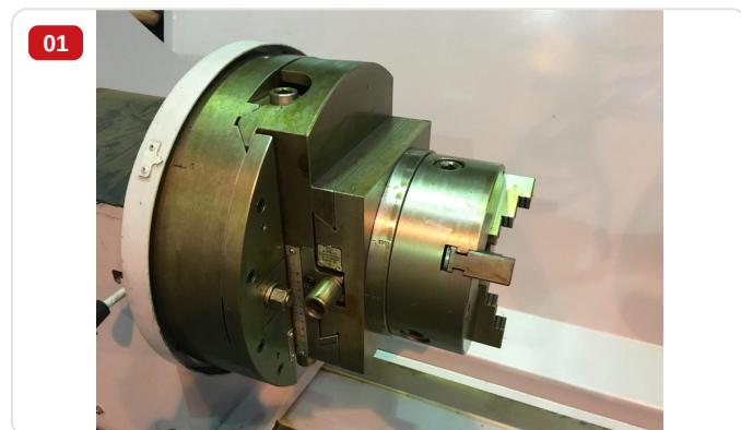
Detalle — Plato universal 8 pulgadas con 3 mordazas de fijación para cigüeñal en rectificadora
