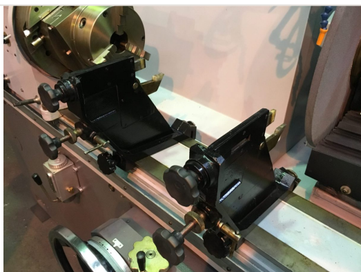
Accesorio normal — Lunetas de apoyo y placas universales de 3 garras fijando cigüeñal en el cabezal portapieza de la rectificadora RVC-1500M
