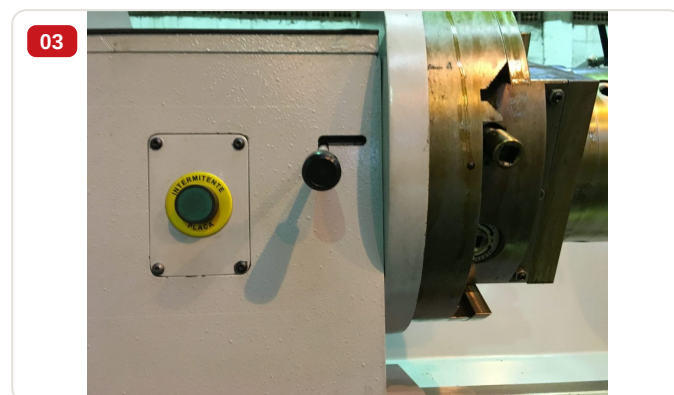
Detalle — Botón para giro intermitente de la placa en panel de control de la rectificadora de cigüeñal RVC-1500M
