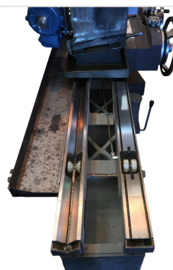
Detalhe — Roletes de lubrificação - barramento com nervuramento interno
