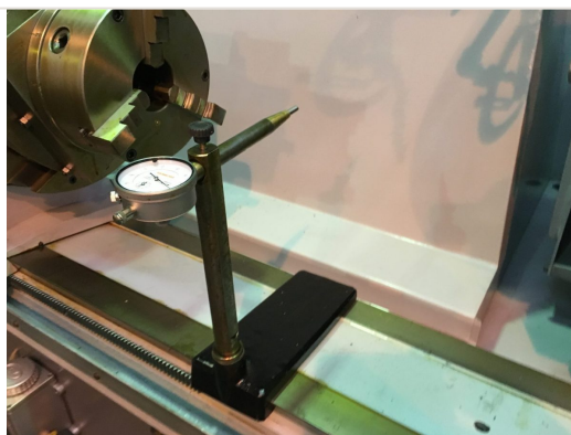
Acessório normal — Dispositivo centralizador
