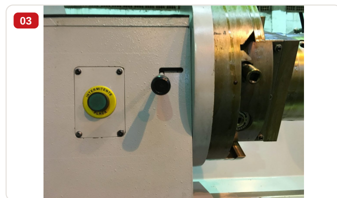
Detalhe — Botão para giro intermitente da placa em painel de controle da retífica de virabrequim RVC-1500M
