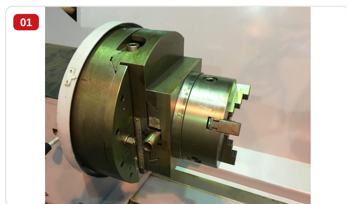
Detalhe — Placa universal 8 polegadas com 3 castanhas de fixação para virabrequim em retífica
