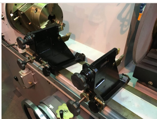
Acessório normal — Lunetas de apoio e placas universais de 3 castanhas fixando virabrequim no cabeçote porta-peça da retífica RVC-1500M
