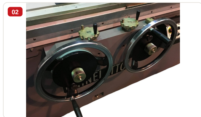
Detalhe — Volantes de avanço da mesa e do cabeçote do rebolo em ferro fundido com punhos centrais
