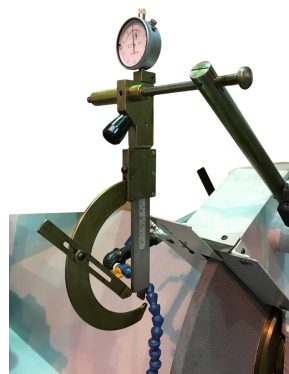
Acessório normal — Dispositivo de medição contínua com relógio comparador em suporte articulado para controle dimensional na retífica RVC-1500M
