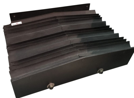
Detalhe — Proteção sanfonada guias cabeçote porta rebolo
